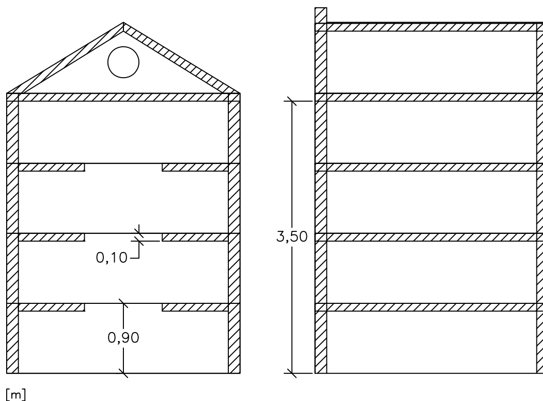
Cortes Transversais
